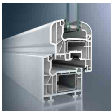
Hohe Basissicherheit: Die Bautiefe von 70 mm und weit innen liegende Beschläge entziehen die Verschlusselemente dem Angriff der Einbrecher.
